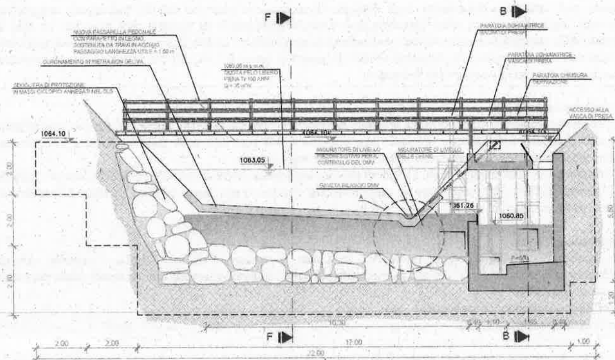
Figura 4 Sezione centrale dell'opera di presa
