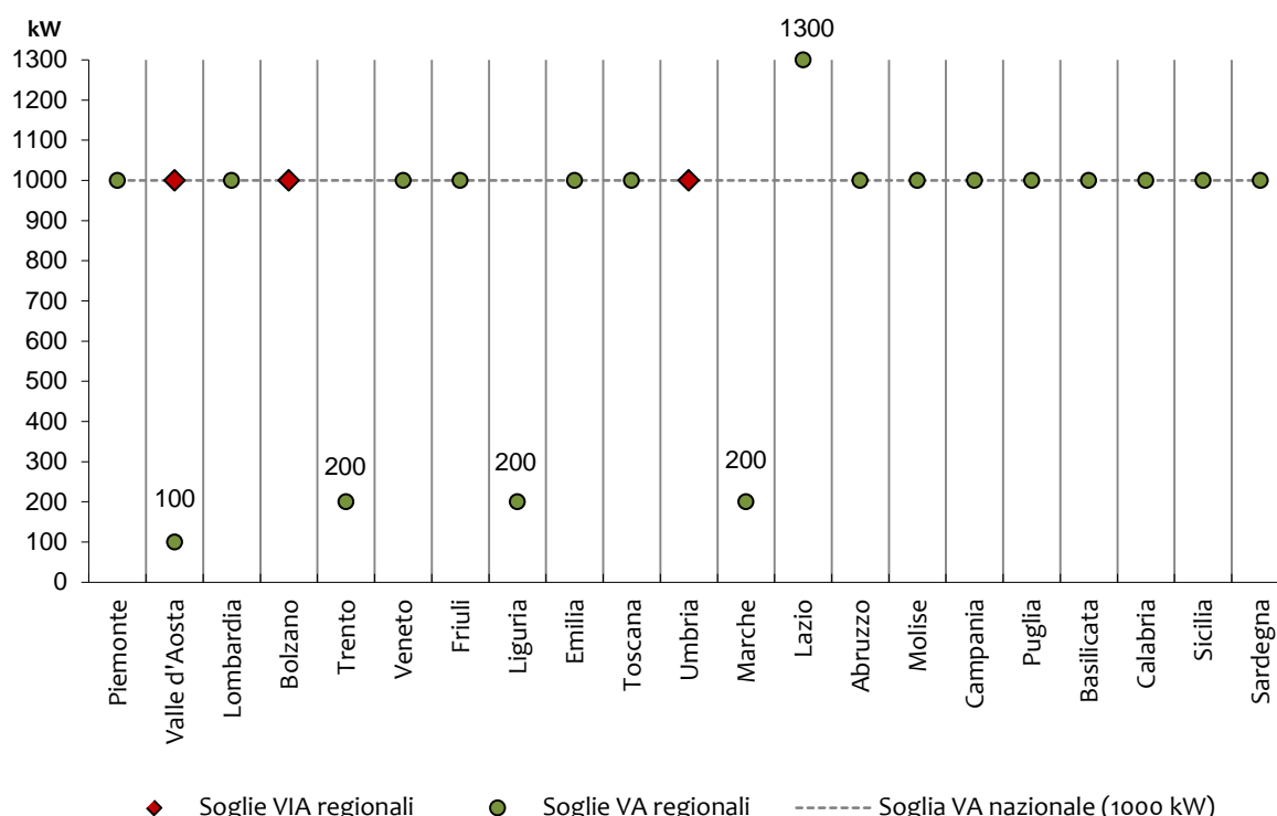
Figura 22. Soglie per le valutazioni ambientali degli impianti fotovoltaici (assetto al 31/12/2018).
