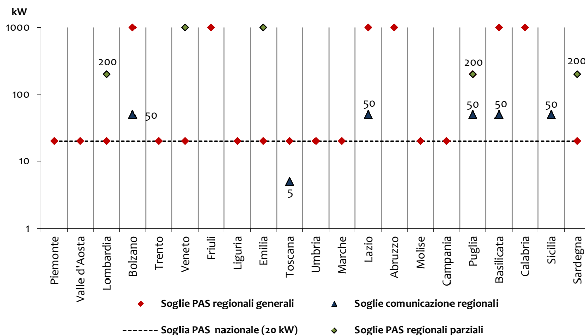
Figura 20. Regimi autorizzativi semplificati per gli impianti fotovoltaici (assetto al 31/12/2018).
