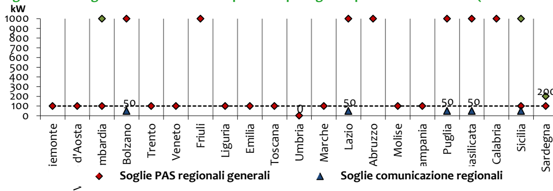
Figura 26. Regimi autorizzativi semplificati per gli impianti idroelettrici (assetto al 31/12/2018).
