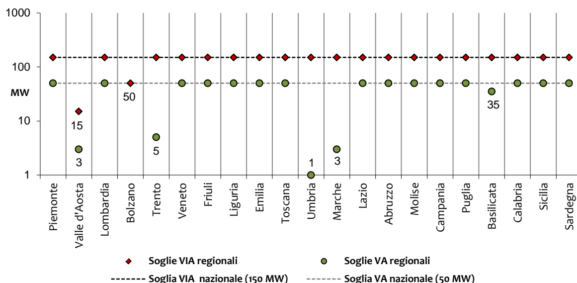
Figura 14. Soglie per le valutazioni ambientali degli impianti alimentati da biomasse e biogas (assetto al 31/12/2018).
