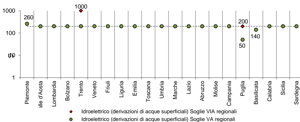
Figura 28. Soglie per le valutazioni ambientali degli impianti idroelettrici con derivazioni di acque superficiali (assetto al 31/12/2018).
