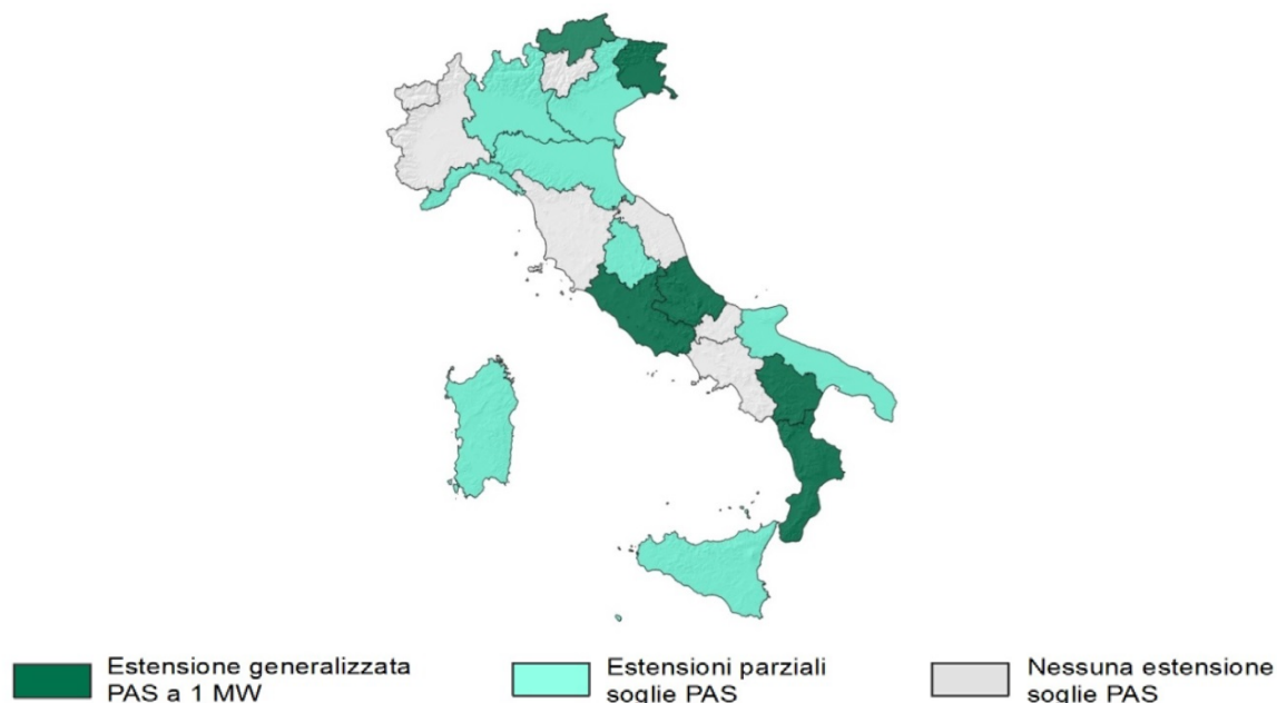
Figura 2. Soglie per l'applicazione della PAS per gli impianti di produzione di energia elettrica alimentati da fonti rinnovabili (assetto al 31/12/2018).
