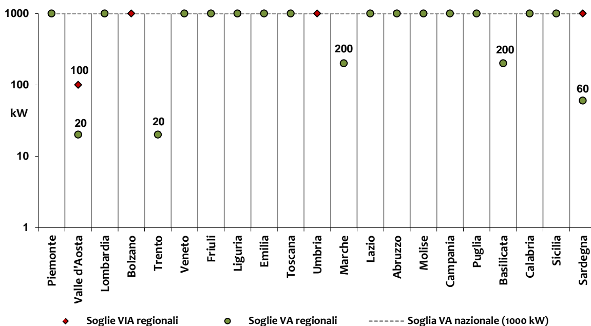
Figura 18. Soglie per le valutazioni ambientali degli impianti eolici (assetto al 31/12/2018).
