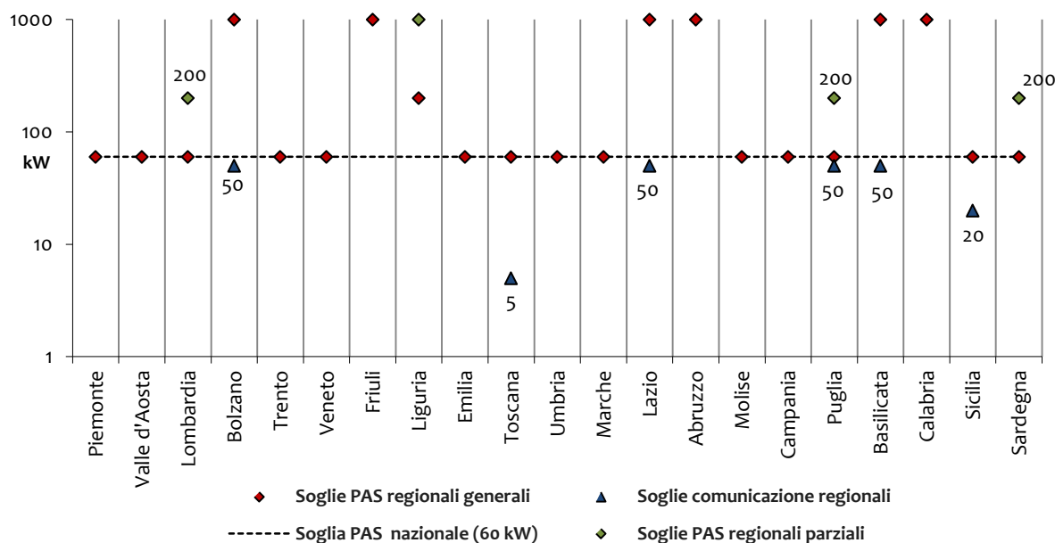
Figura 16. Regimi autorizzativi semplificati per gli impianti eolici (assetto al 31/12/2018)
