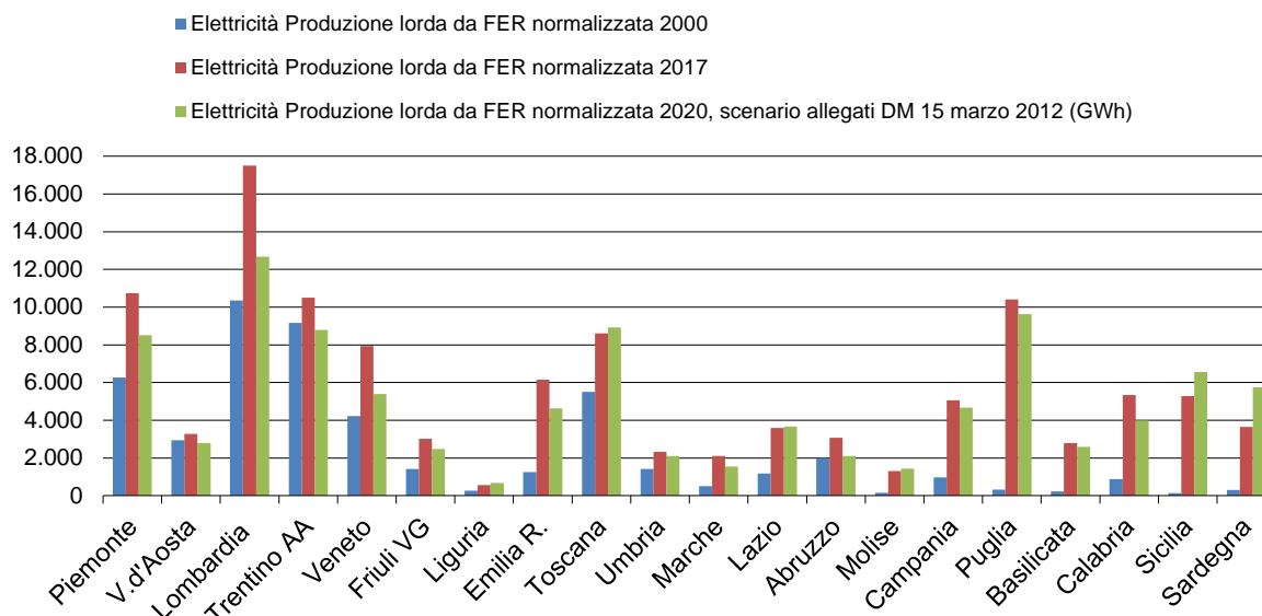
Figura 10. Energia elettrica: produzione lorda da rinnovabili (eolico e idroelettrico normalizzati) negli anni 2000*, 2017 e obiettivi regionali 2020 (GWh)
