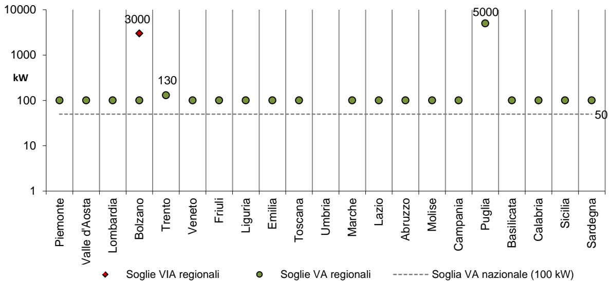
Figura 29. Soglie per le valutazioni ambientali degli impianti idroelettrici (assetto al 31/12/2018).
